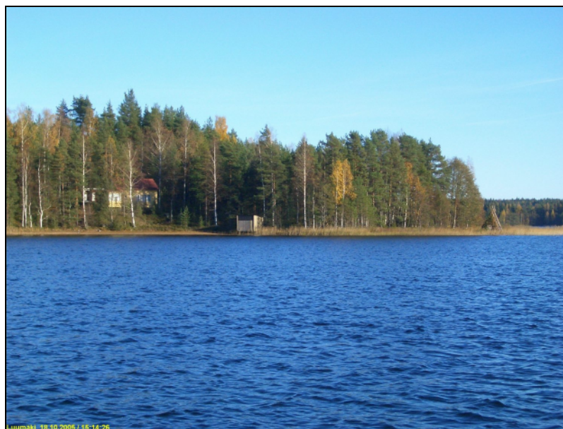
Naimasaaren lounaispää, jonka rantavedestä ja rannalta kvartseja. Kuvattu lännestä.
